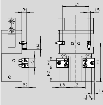
DASI-B10-25-S8
