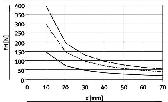
HGRT-20-A
