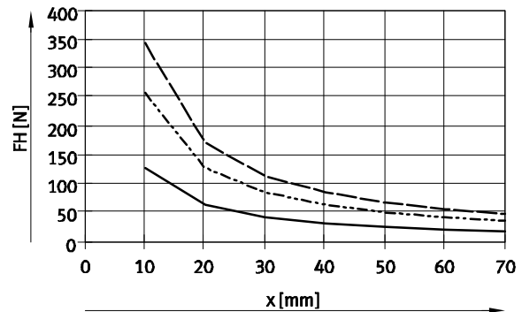
HGRT-20-A
