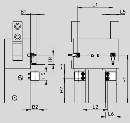
DASI-B10-40-S12
