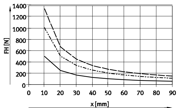
HGRT-32-A
