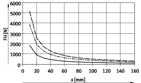
HGRT-50-A
